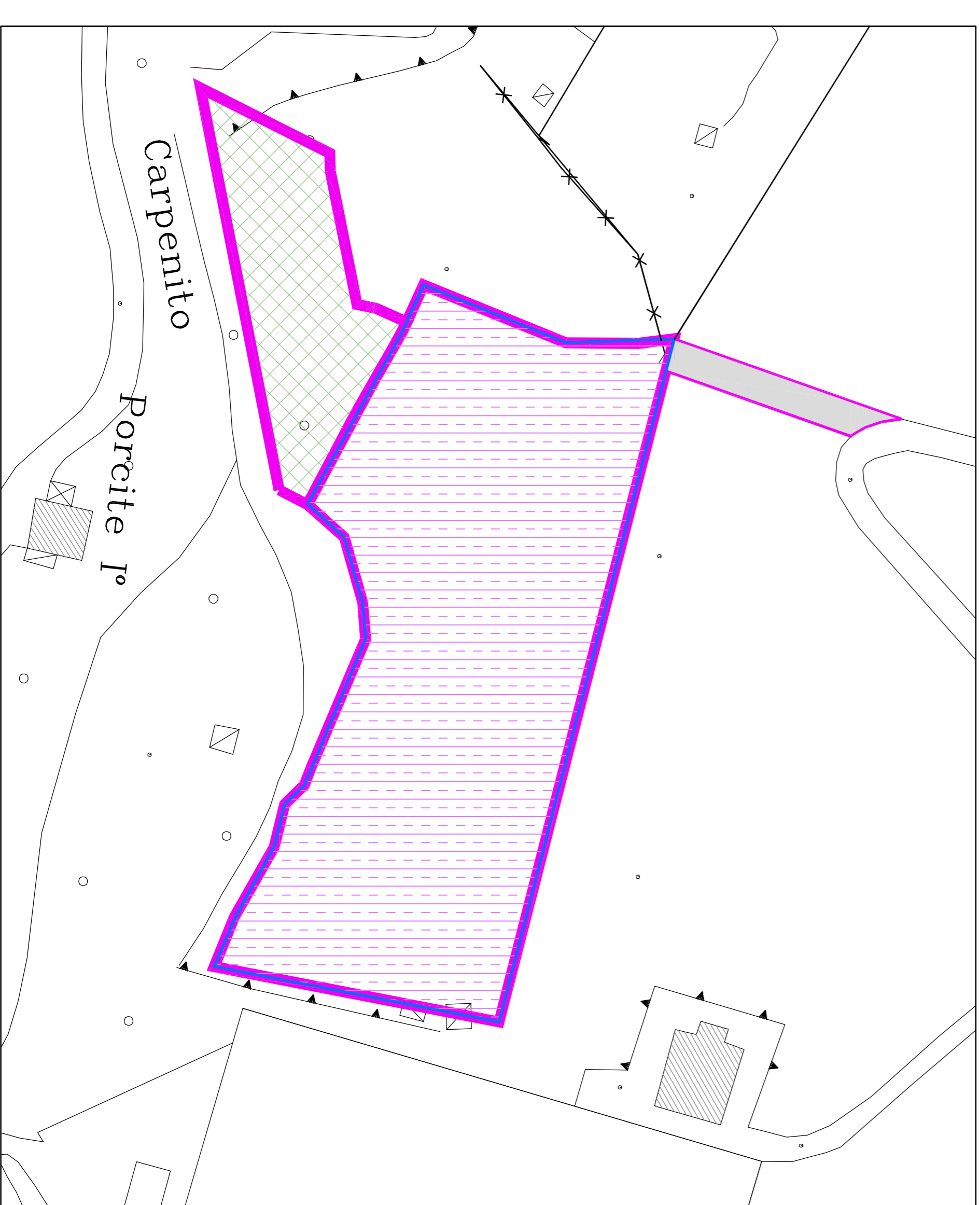
Riferimento planimetrico
